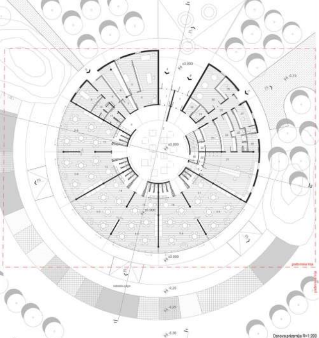
Osnova prizemlja Rn=1:200
