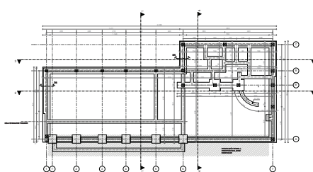
osnova temelja
