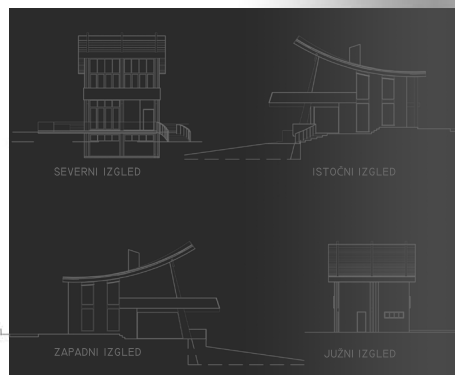
OBJEKAT U OKRUŽENJU
