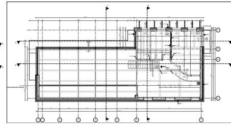
osnova sprata
