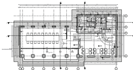
osnova prizemlja
